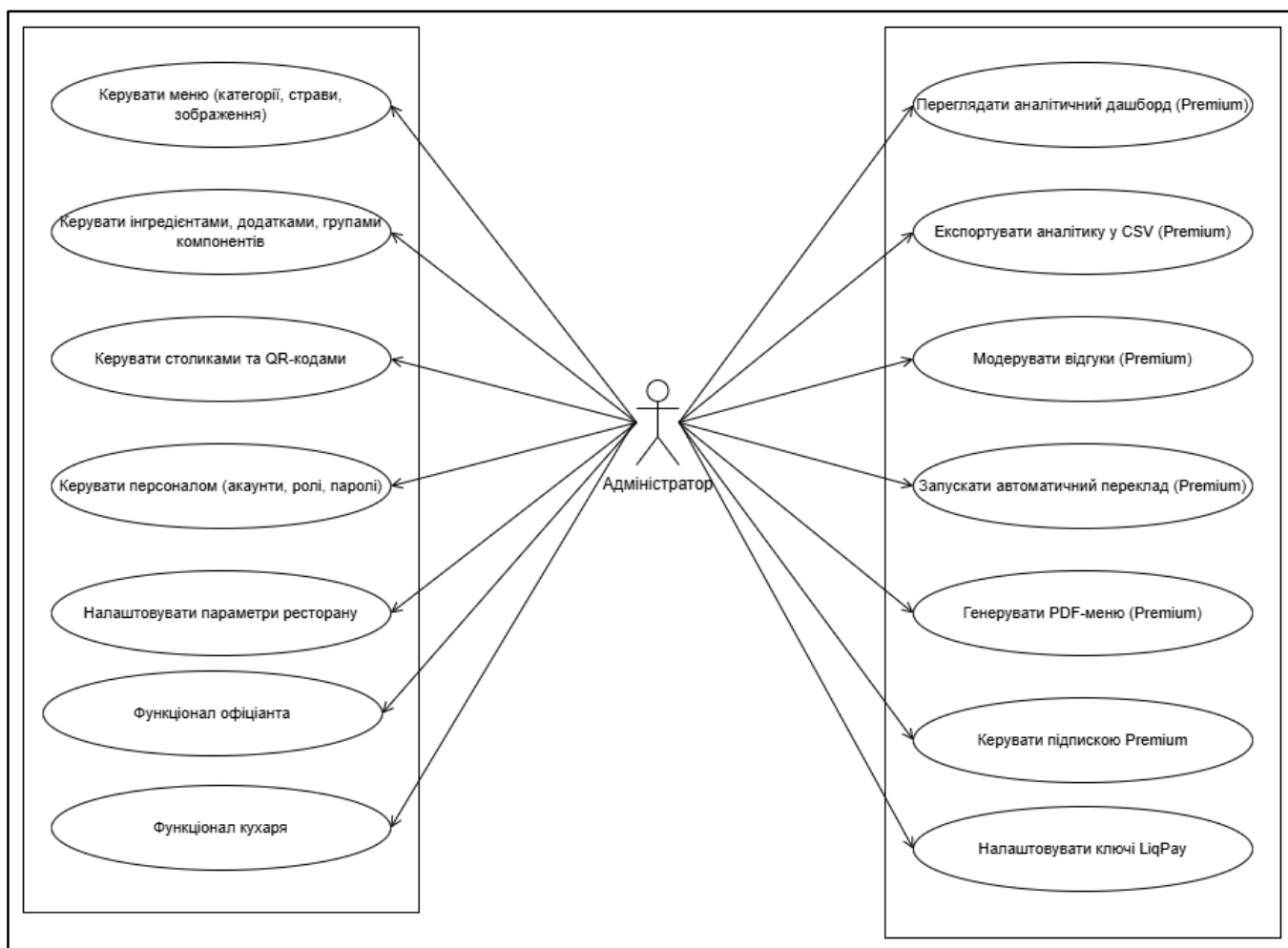
Рисунок 3.4 – Use case діаграма ролі «Адміністратор»
