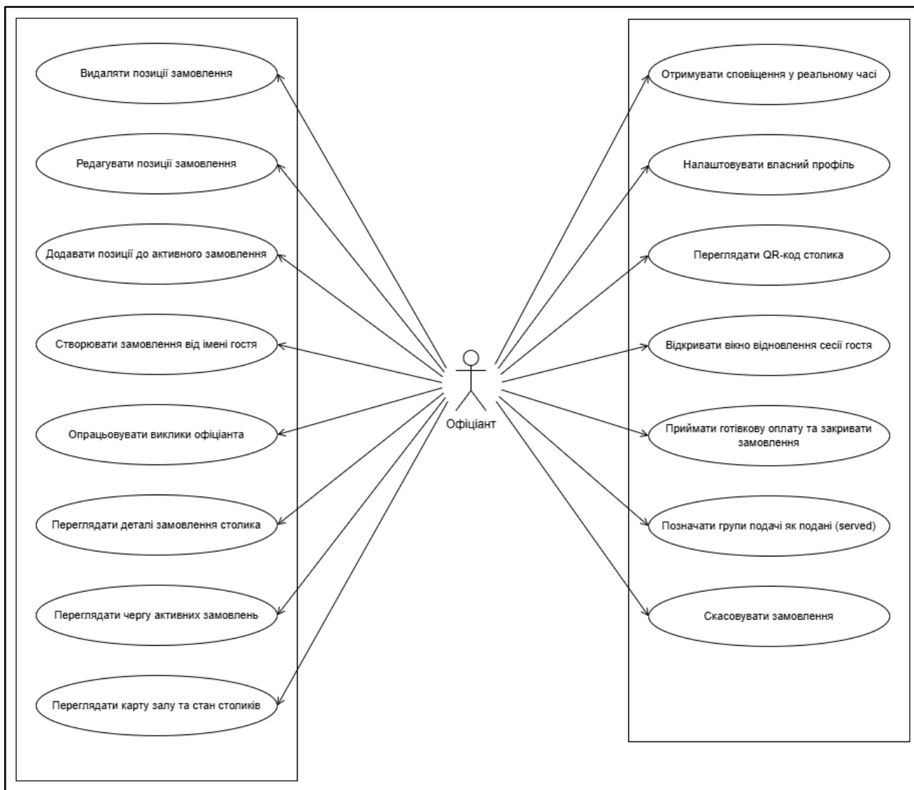
Рисунок 3.2 – Use case діаграма ролі «Офіціант»
