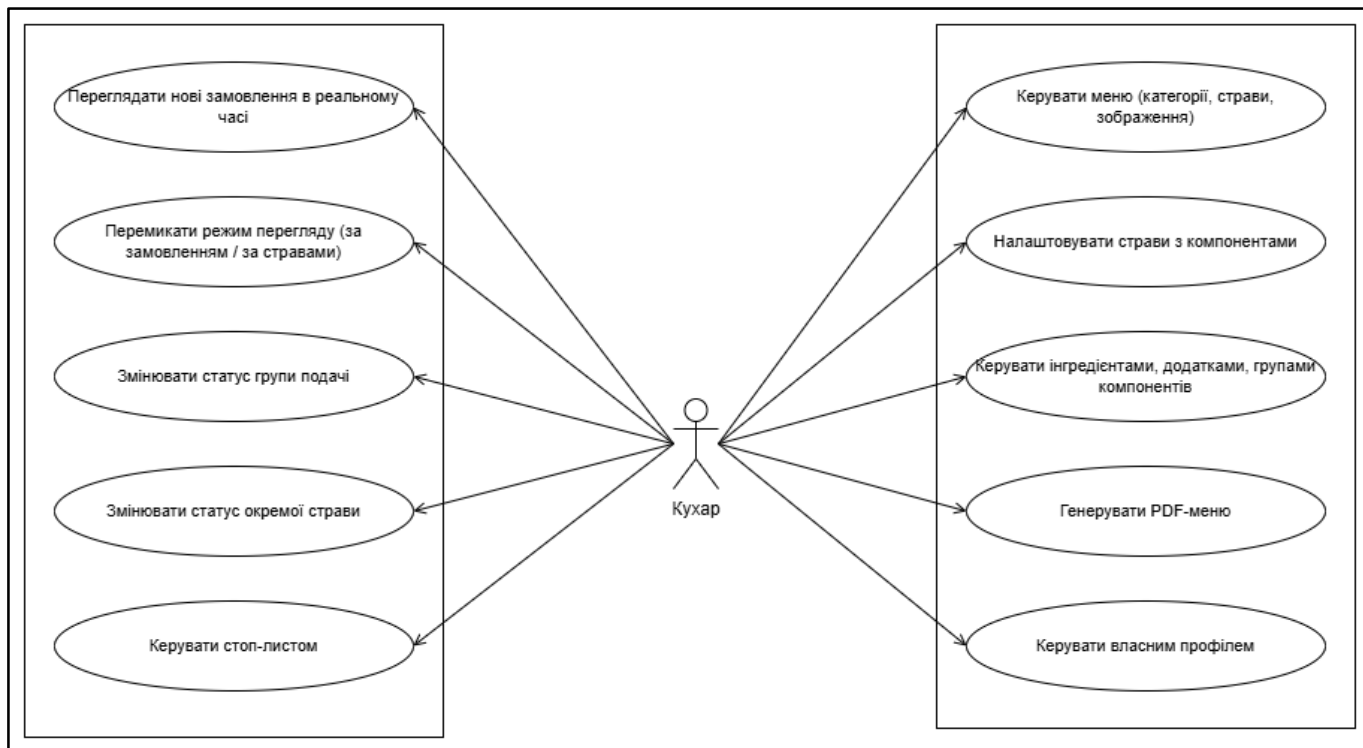
Рисунок 3.3 – Use case діаграма ролі «Кухар»
