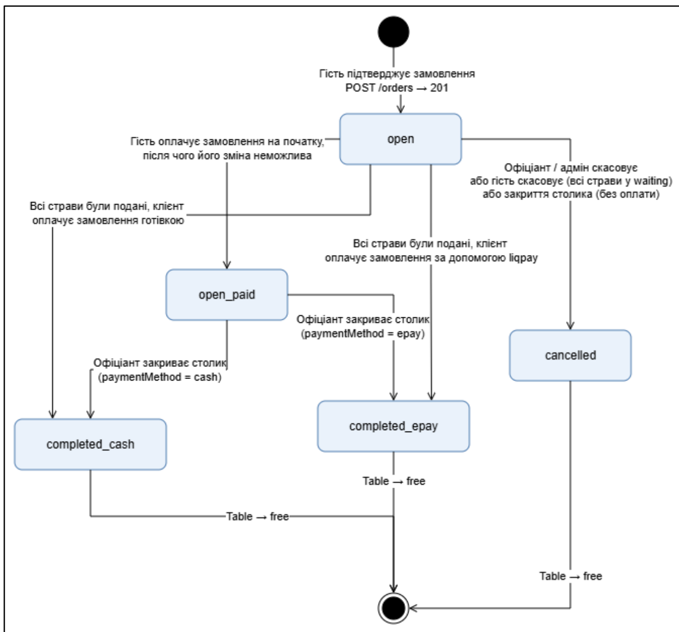
Рисунок 3.5 – Діаграма станів замовлення (Order State Diagram)
