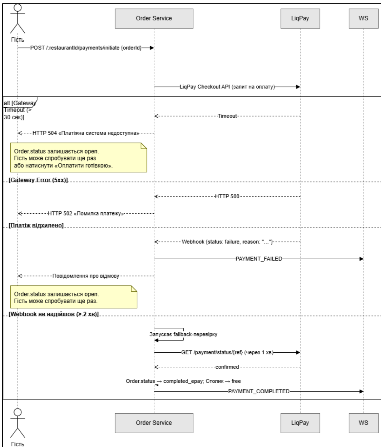
Рисунок 3.7 – Sequence-діаграма обробки помилок платіжного шлюзу та fallback-механізму
